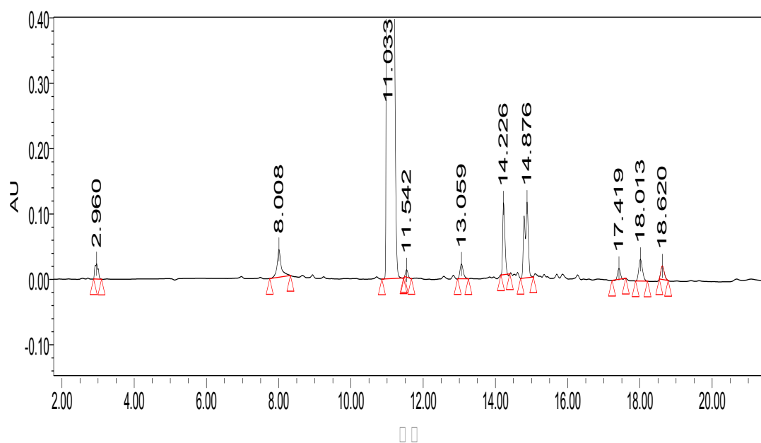
图 1 样品色谱图
